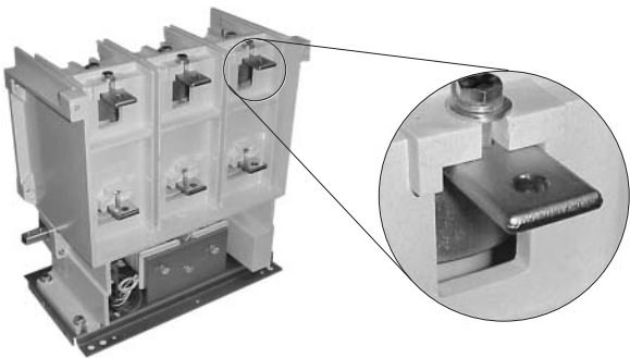
Lug Terminal
